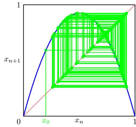
100 iterazioni con a = 3.7 , x_0 = 0.2
