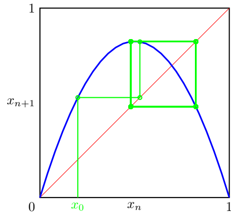
100 iterazioni con a = 3.3 , x_0 = 0.2
